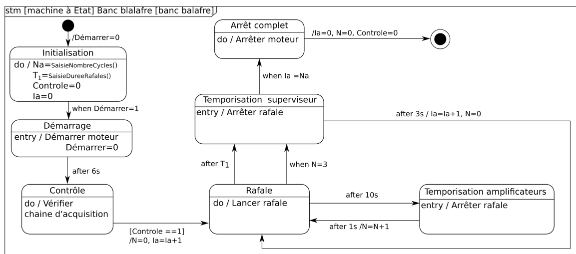
FIGURE 23 – Diagramme d'état à modifier pour prendre en compte une anomalie détectée pendant la phase de contrôle.
