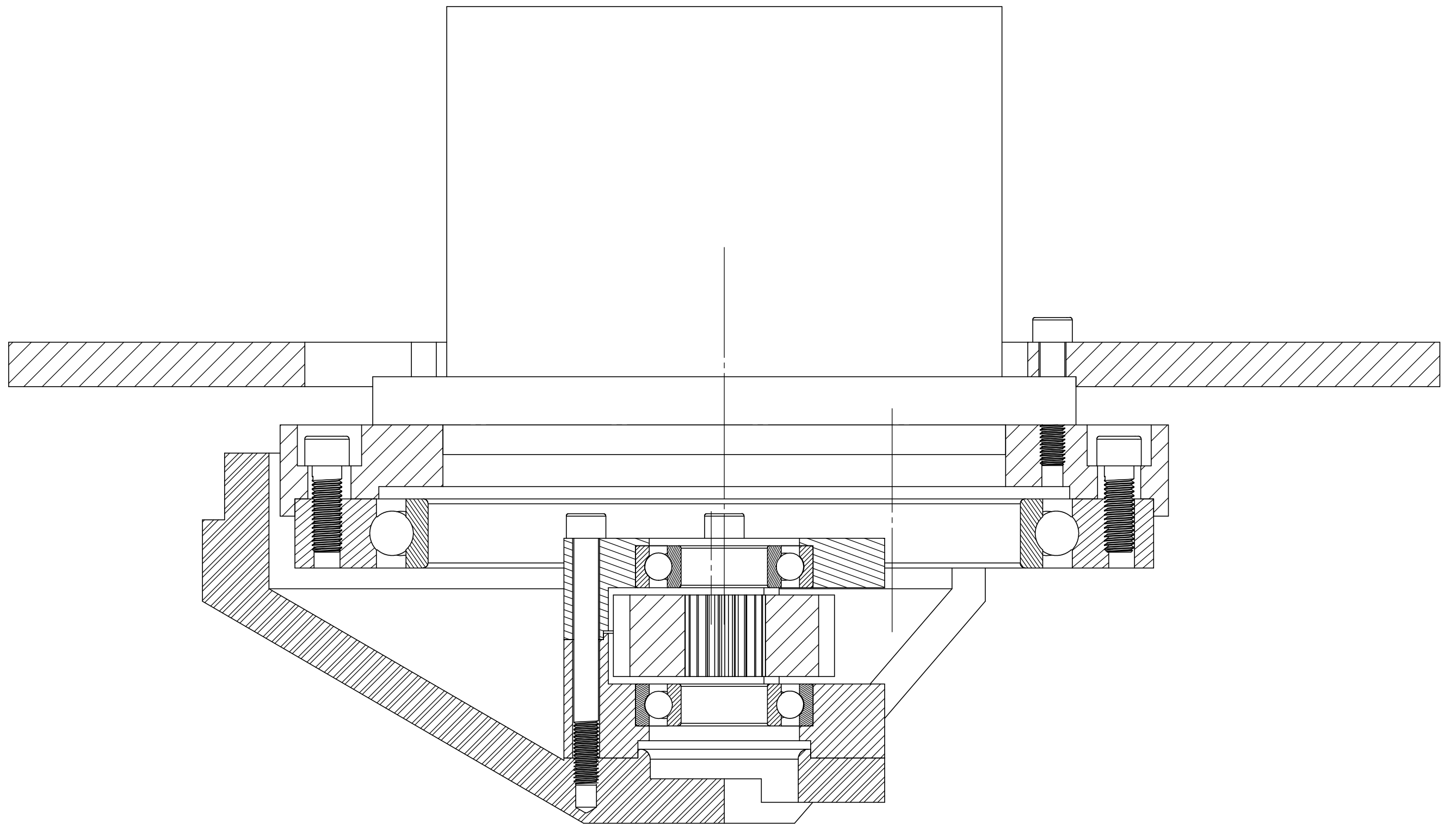
COUPE A-A
